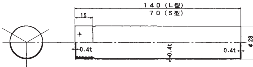
図 4.3.6 簡易照射筒設備用キャプセル (アルミニウム製)
