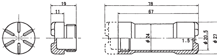
図 4.3.7 気送管照射筒設備用キャプセル (ポリエチレン製)
