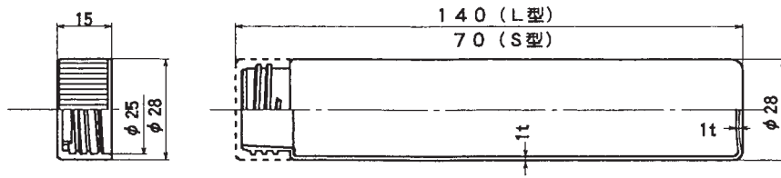
図 4.3.5 簡易照射筒設備用キャプセル (ポリエチレン製)
