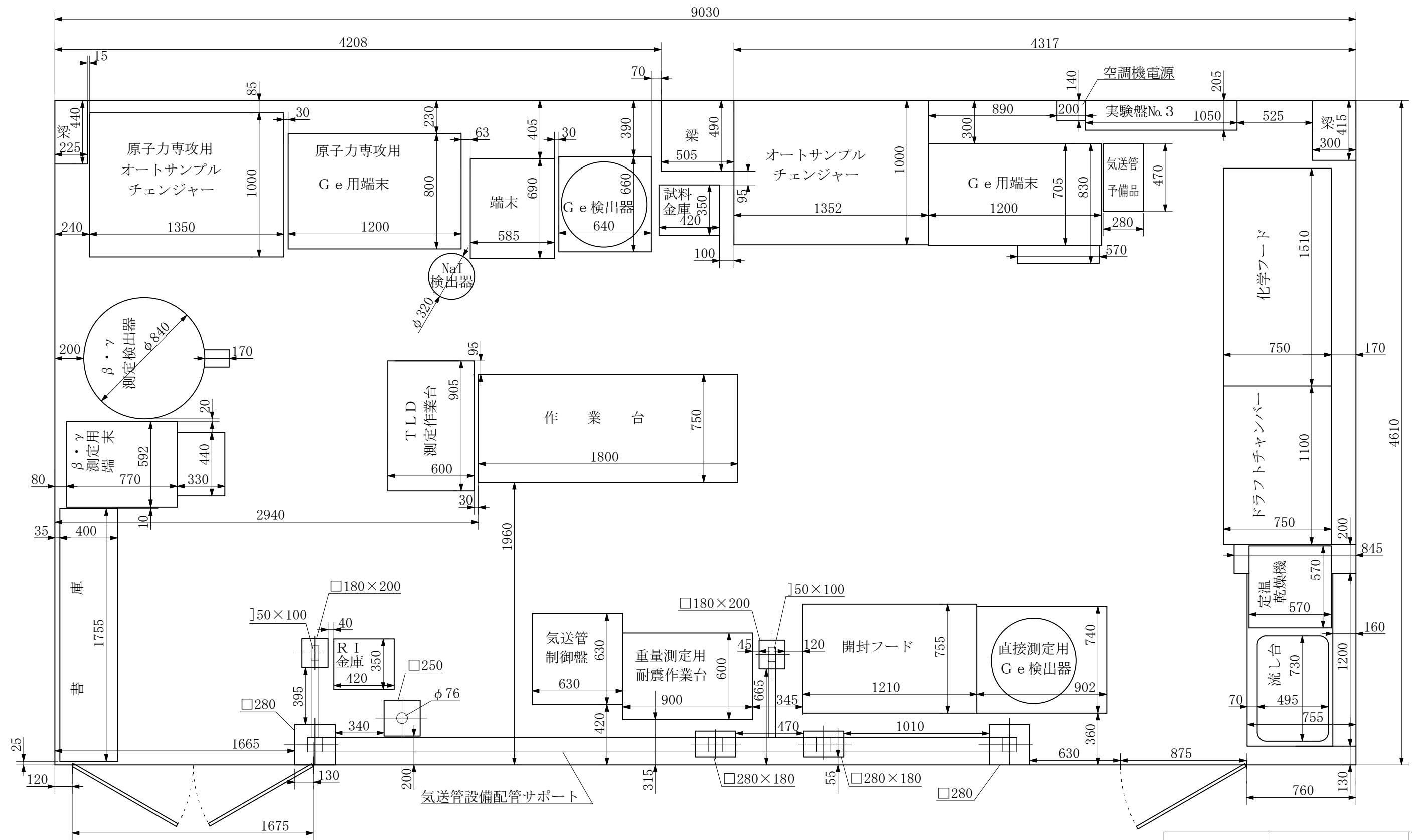
ホット実験室機器配置寸法図
